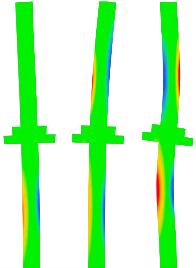
Differenzierter Lasteinfluss an Stützen im Lastfall «Erdbeben».
