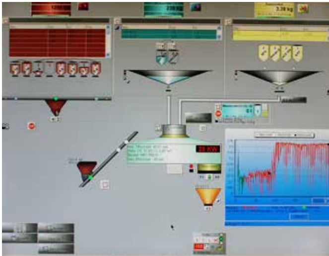
Prozessgesteuerte Betonanlagen mit Protokollhinterlegung.
