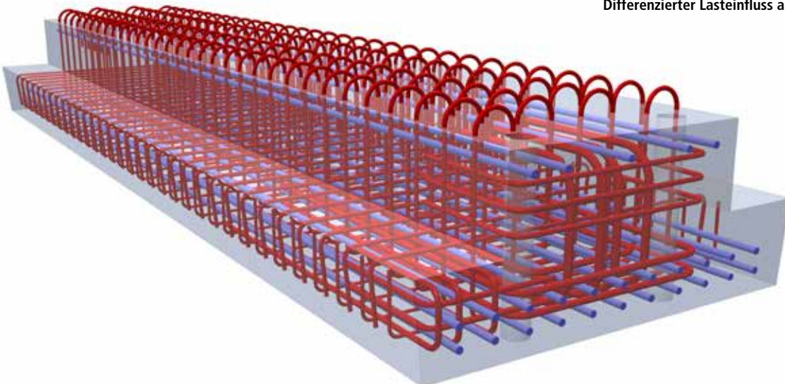
Prüflayout eines hoch vorgespannten und bewehrten Hutträgers.
